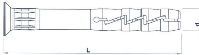
FX-N-..L.. sleeve
